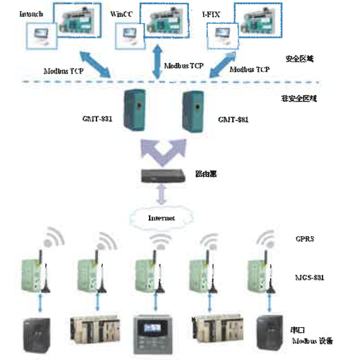
PLC远程监控(速联A/B)
