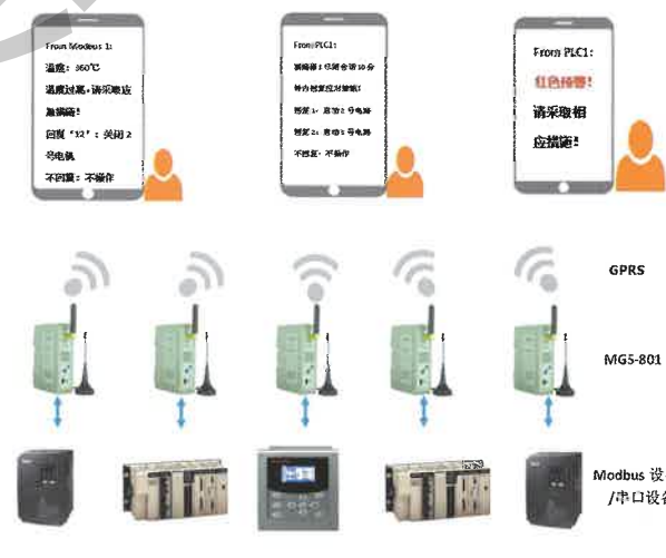
MGS-801短信报警
