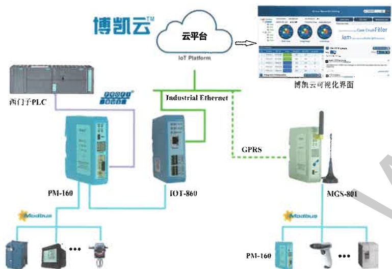
网关与云端监控/数采整体方案
